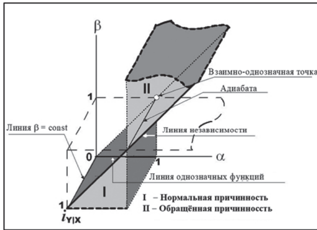
Рис. 2. Энтропийная диаграмма типов взаимосвязи процессов.
