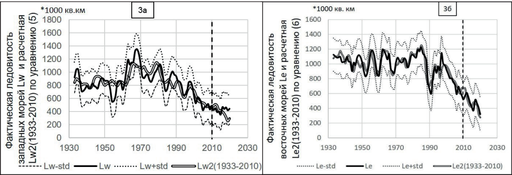
Рис. 3. Фактические Lw, Le (толстые черные линии) и рассчитанные Lw2_{(1933-2010)}, Le2_{(1933-2010)} (тонкие двойные линии) площади льдов в августе в западных (а) и в восточных (б) морях Арктики для периода с 1933 г. по 2010 г., ограниченного на рисунках вертикальной штриховой линией. Пунктирными линиями нанесены значения ледовитости минус и плюс стандартное отклонение ( Lw-std, Le-std и Lw+std, Le+std ).
