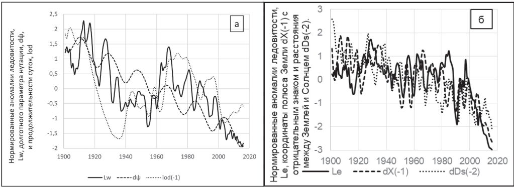
Рис. 1. Временные серии аномалий трехлетних, скользящих нормированных на средне-квадратическое отклонение ледовитости Lw, Le в западном секторе (а) и восточном секторе Арктики (б), а также астрогеофизических характеристик: долготного параметра наклона оси Земли, dψ; продолжительности суток, lod; координаты полюса Земли, dX(-1) с отрицательным знаком, и аномалии расстояния между Землей и Солнцем, dDs(-2).
