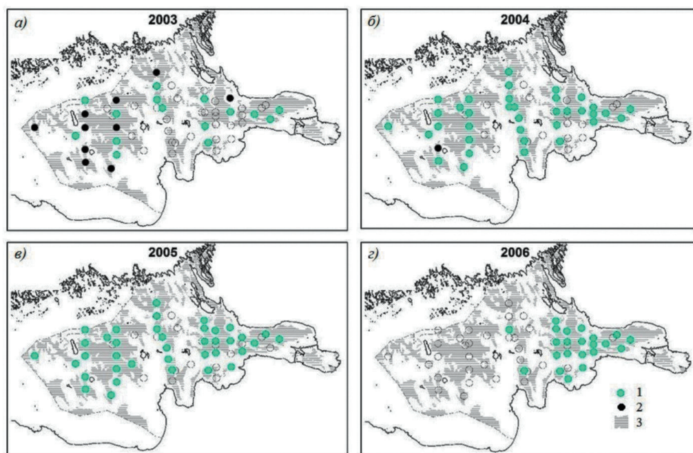
Рис. 3. Карты пространственной изменчивости содержания растворенного кислорода в придонных водах по данным мониторинговых наблюдений РГГМУ
