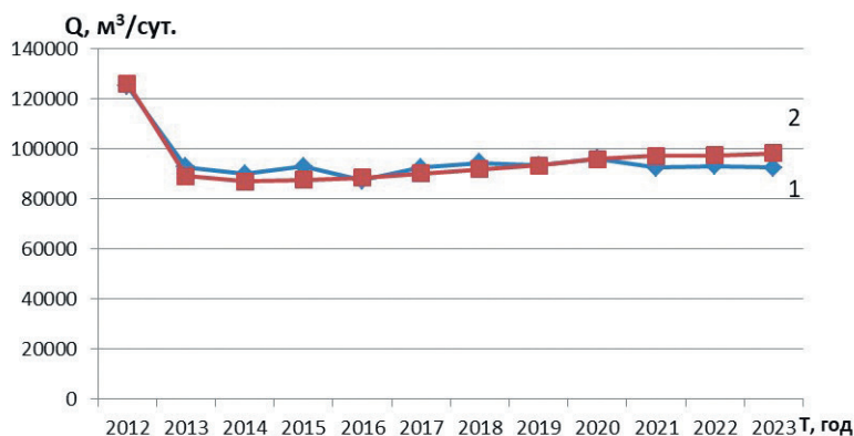
Рис. 5. Спрогнозированные по модели водосбора (1) и рассчитанные с помощью геофильтрационной модели (2) значения среднегодового водопритока к карьеру, вскрывшему палеогеновые отложения, при отсутствии воздействия дренажной системы.
