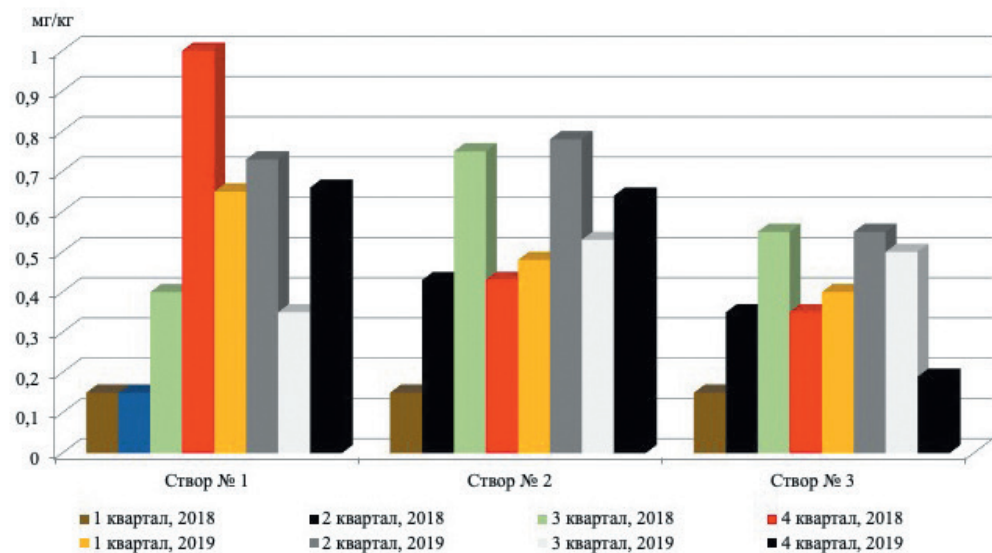
Рис. 6. Концентрация кадмия в донных отложениях за исследованный период.
