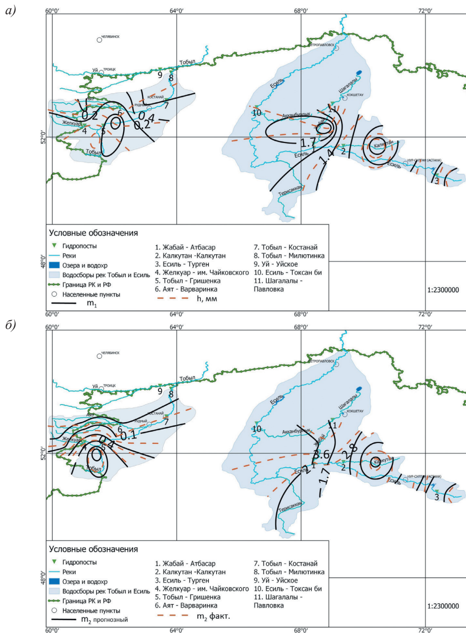
Рис. 2 (начало). Пример карт распределения фактических и прогнозных первого ( a , b ) и второго ( b , c ) статистических начальных моментов через 5 суток ( a , b ) и 25 суток ( b , c ) от даты начала прогноза (прогноз давался с суточным шагом).
